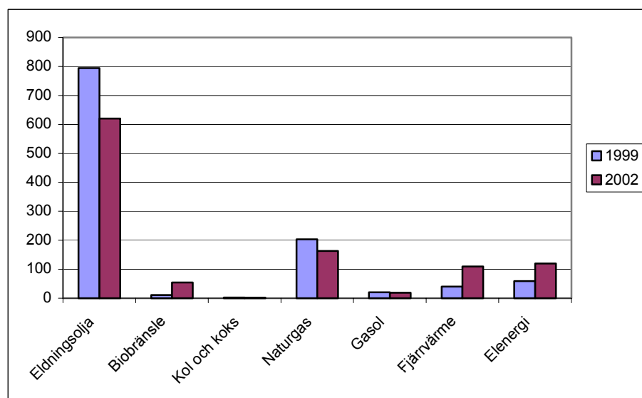
Diagram 8. Energiförbrukning i växthus i 1000-tal MWh efter typ av värmekälla, 1999 och 2002.
